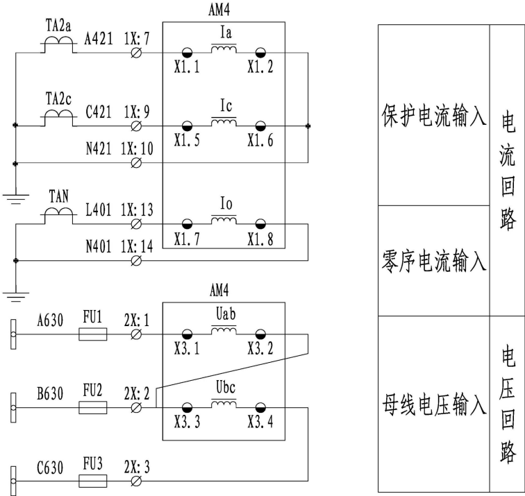
图 5.2 2PT 2CT 接线方法 Figure 5.2 2PT 2CT Wiring method
