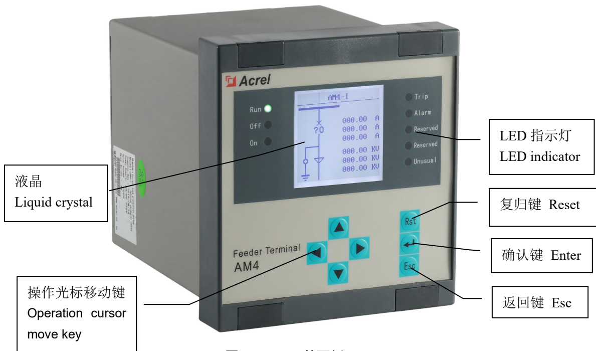
图 3.1 AM4 前面板
