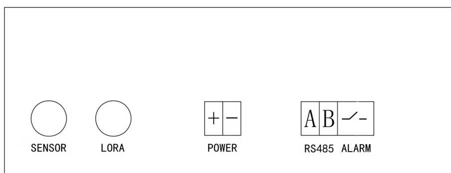
图 1.7 APD100 端子图
