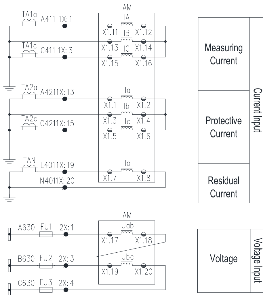
Fig 5.2 2PT&2CT Wiring
